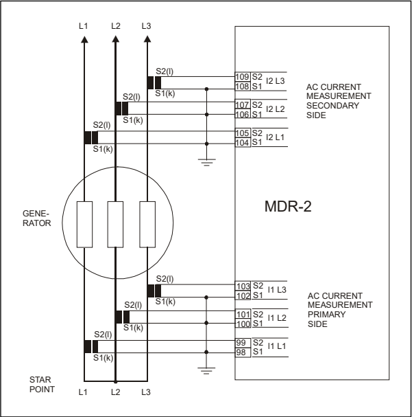
原理图
