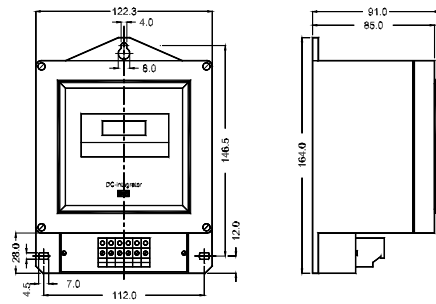
DCF-Q96 (Aufbau)
