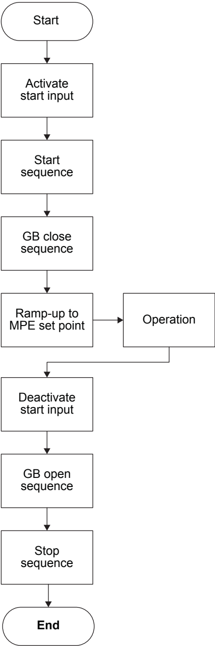
主电源输出流程图
