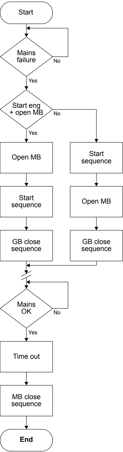
自动电源故障流程图
