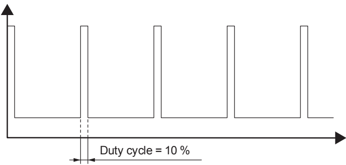
示例：10% 占空比
