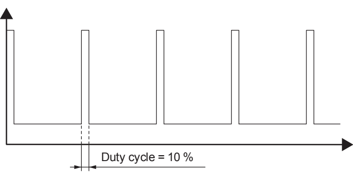
图 6.2 示例：10% 占空比
