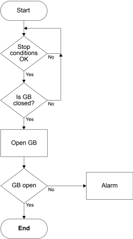
Diagrama de flujo de secuencia de apertura del GB
