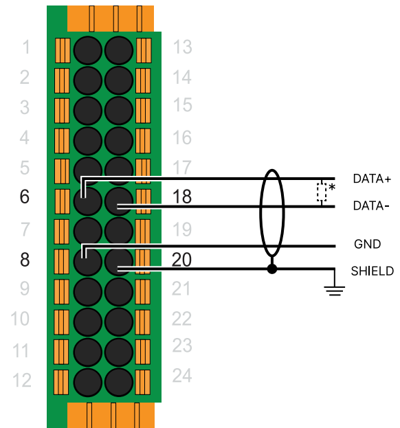
RS-485 port 2*
