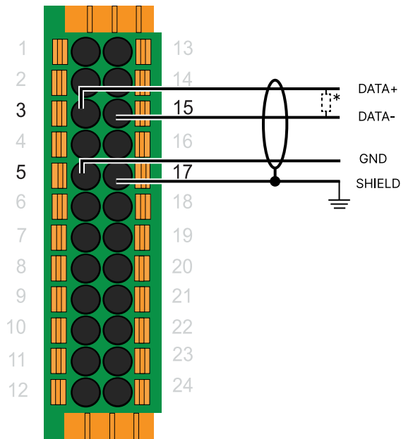
RS-485 port 1*
