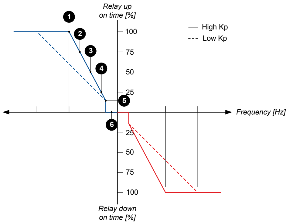
图 8.3 继电器动作（基于周期时间结束时的测量值）
