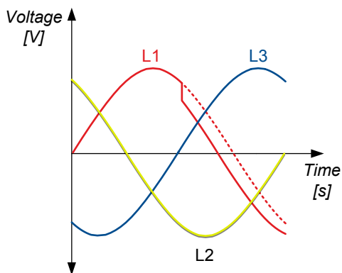
图 5.2 仅 L1 相出现矢量偏移
