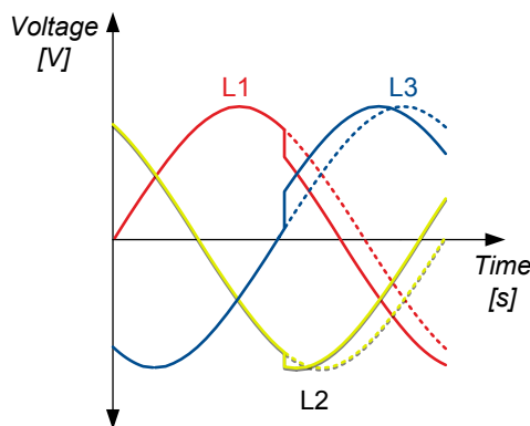
图 5.3 所有相都出现矢量偏移
