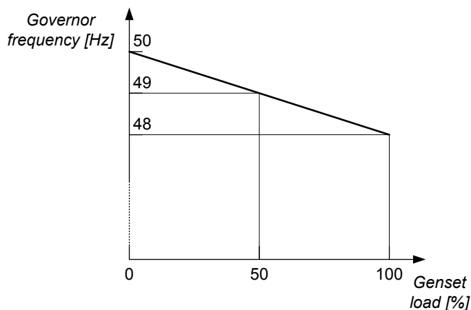
图 8.4 频率下垂为 4% 的发电机组的频率下垂曲线示例
