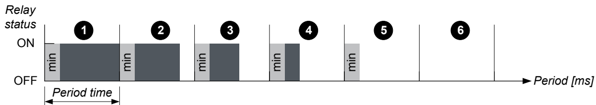
图 8.3 继电器动作（基于周期时间结束时的测量值）
