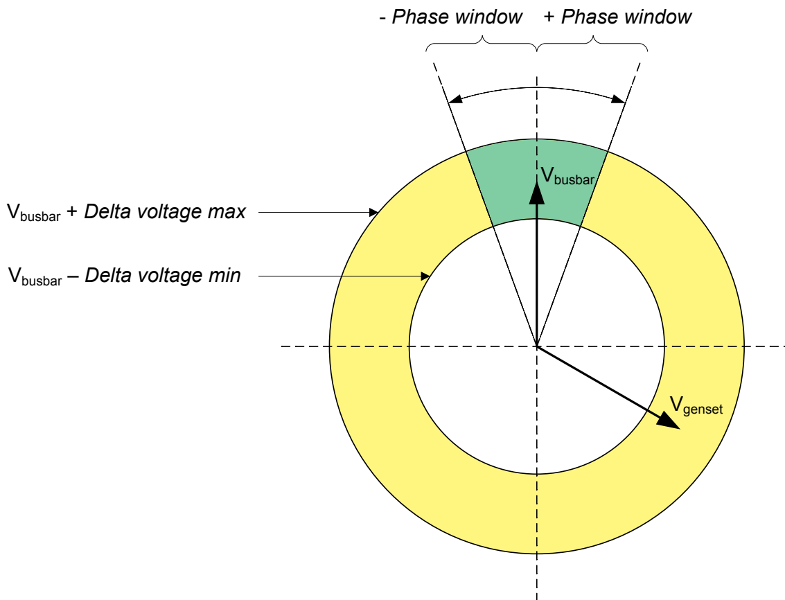
图 7.2 静态同步的电压和相位差
