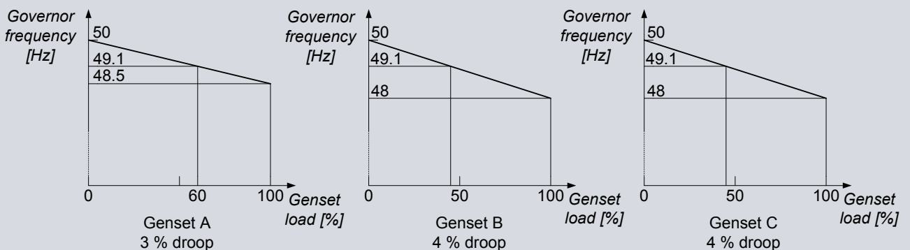
图 8.6 发电机组 A、B 和 C 的下垂曲线
