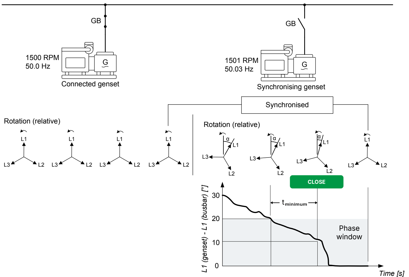
图 7.1 静态同步原理
