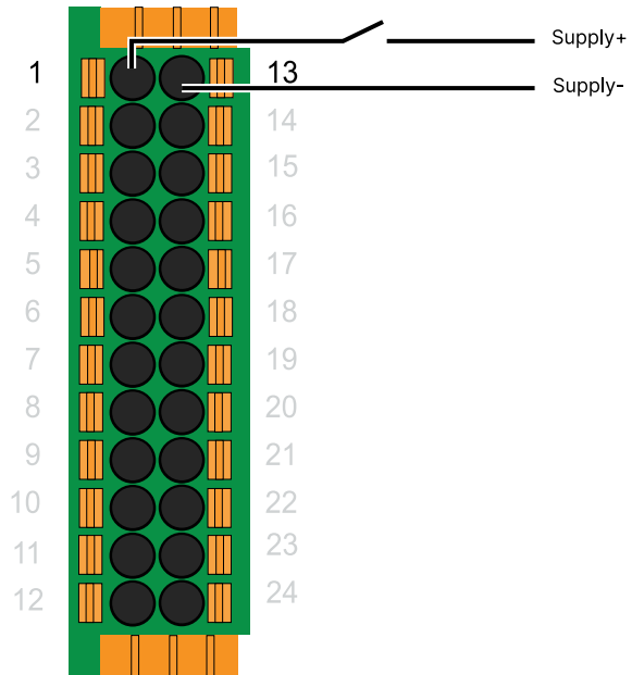
Entrada digital
