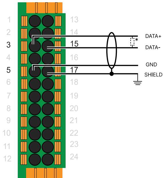
RS-485 porta 1*
