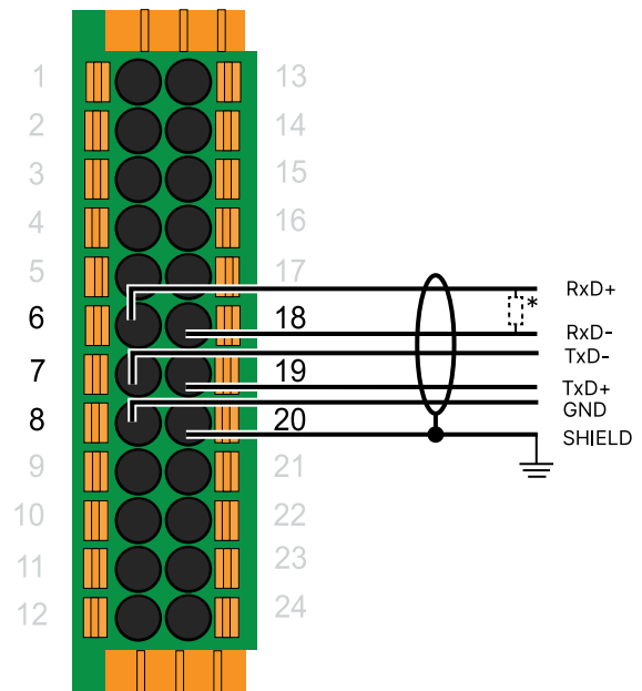
RS-422 porta 2*
