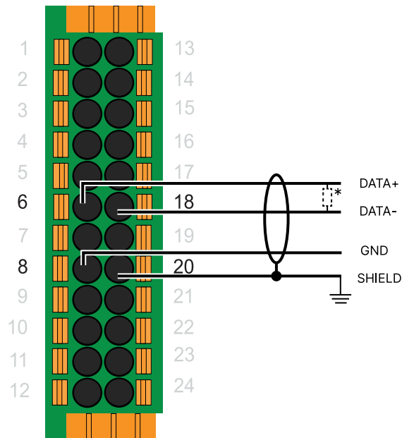
RS-485 porta 2*
