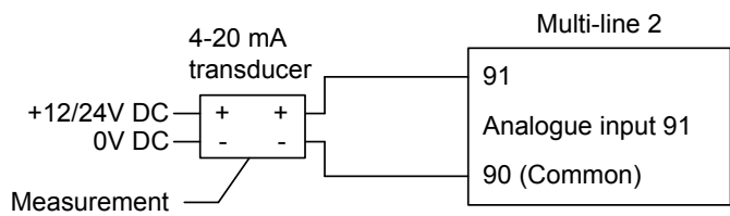
有源变送器（4 至 20 mA）
