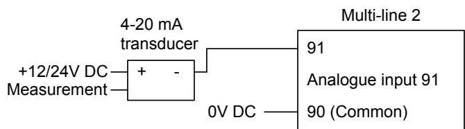
无源变送器（4 至 20 mA）
