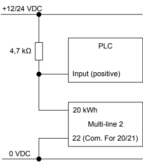
与 PLC 连接：
