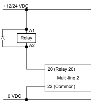
继电器输出：
