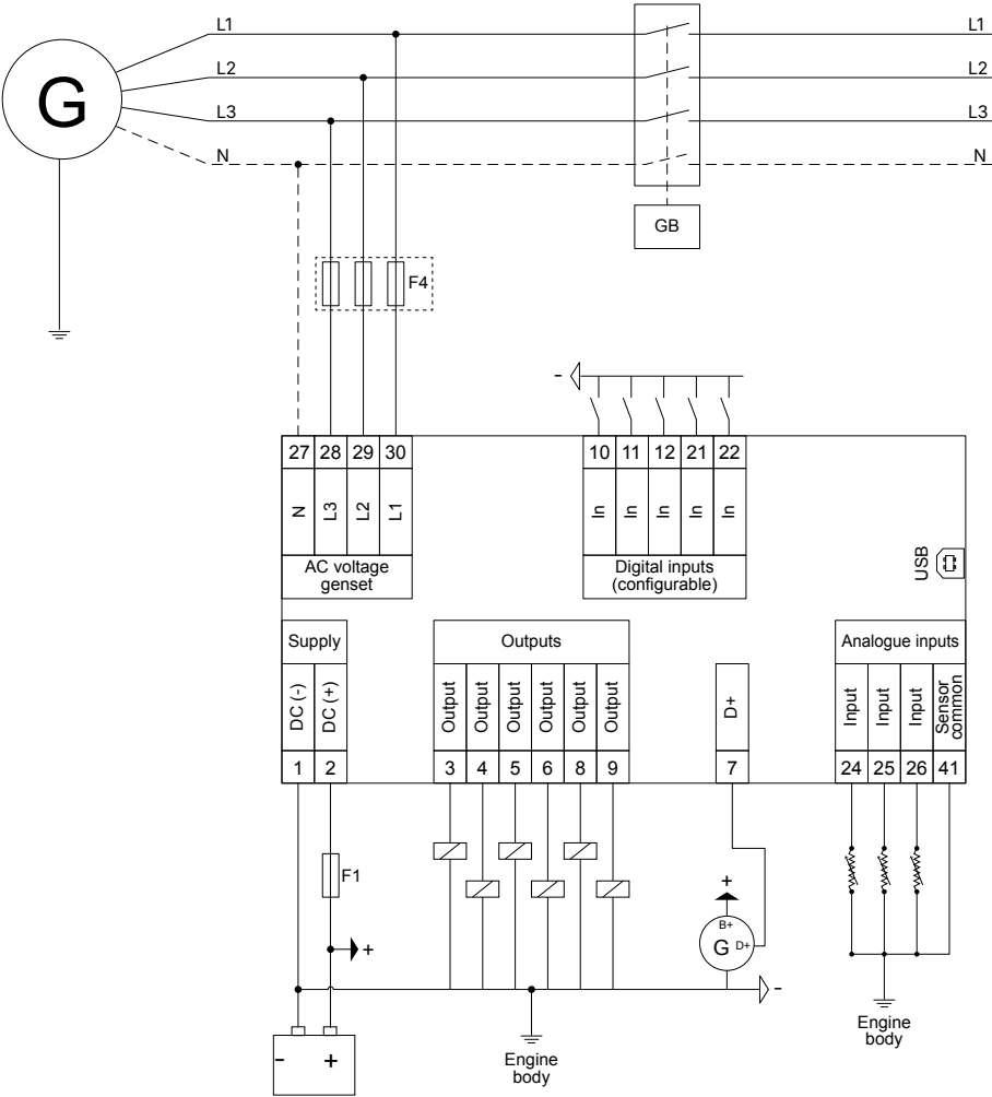
图 4.1 SGC 110 典型接线图
