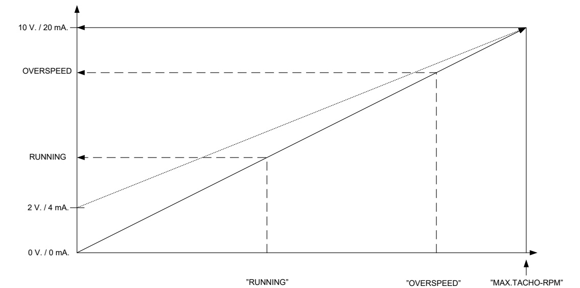
用于缩放模拟量运行中反馈信号的可调设定点的意义
