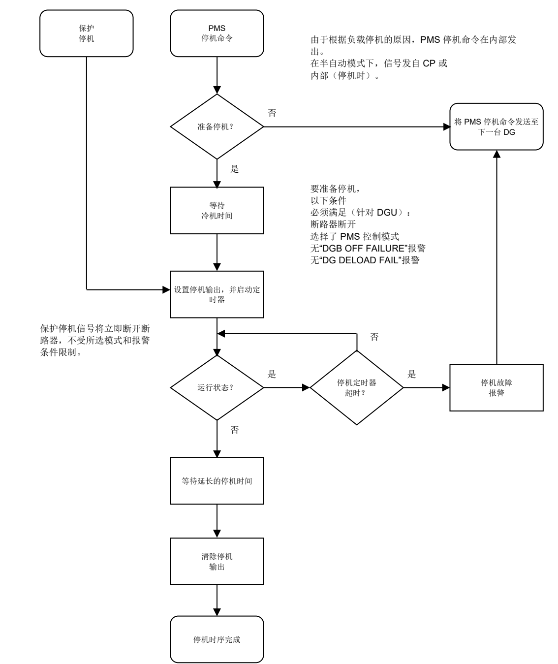
自动停机时序流程图
