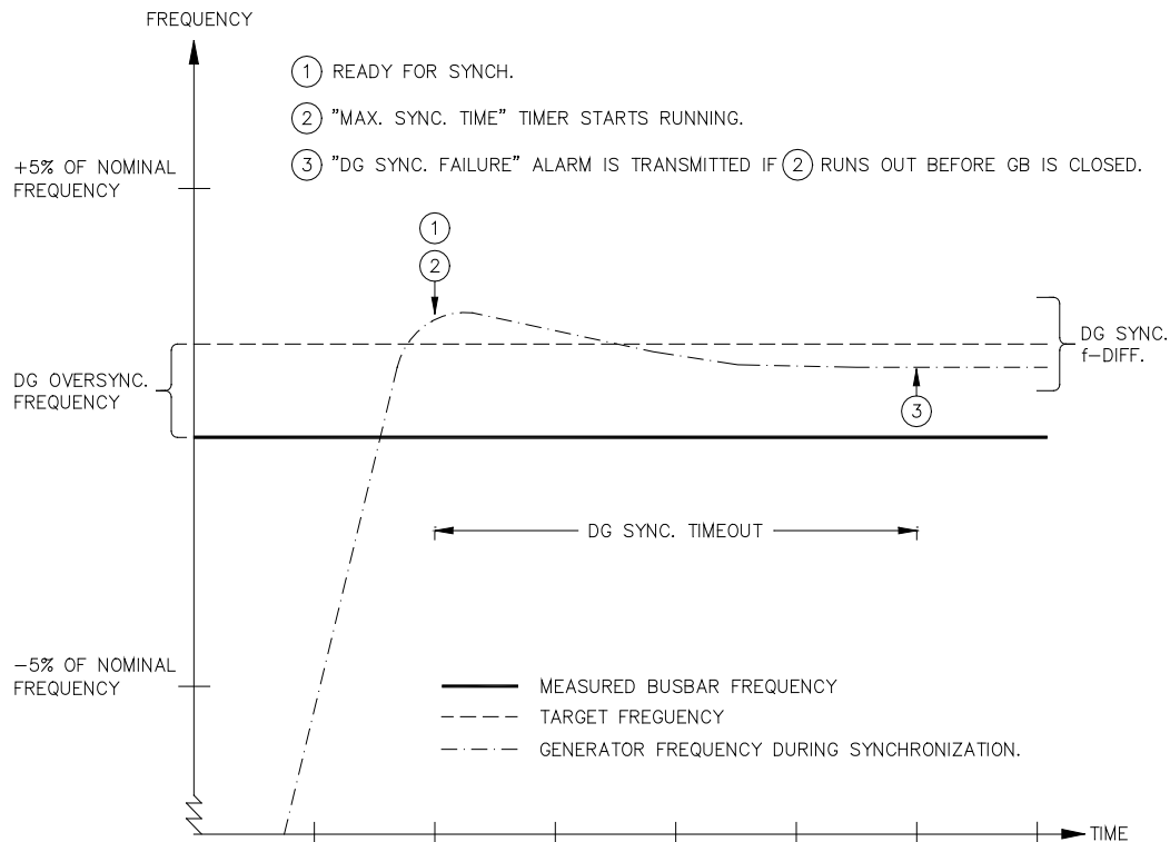
用于动态同步控制的可编程延时和设定点
