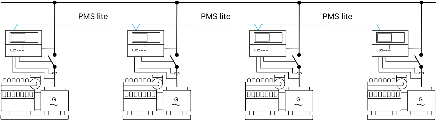
轻型 简单并机 PMS（最多 127 个柴发电机组）
