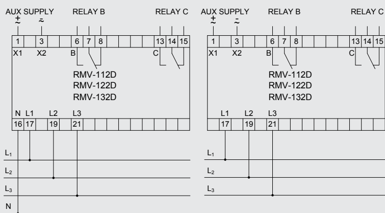
Stern-Schaltung
