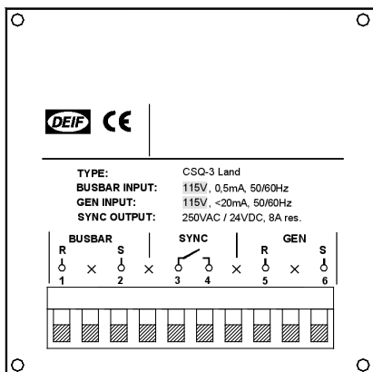
Version terrestre
